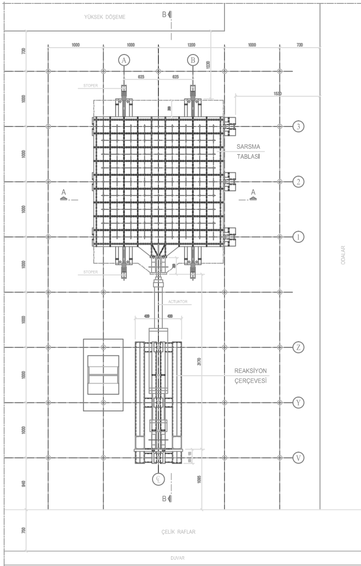
YERLEŞİM PLANI 1/20
