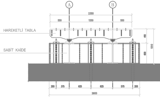
A - A KESİTİ 1/20
