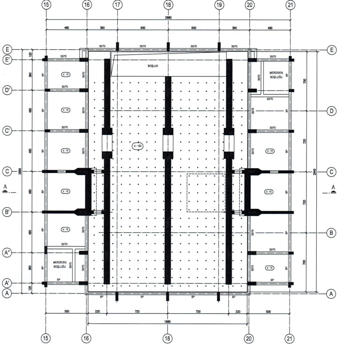
BODRUM KAT TAVANI RÖLÖVE KALIP PLANI 1/100
