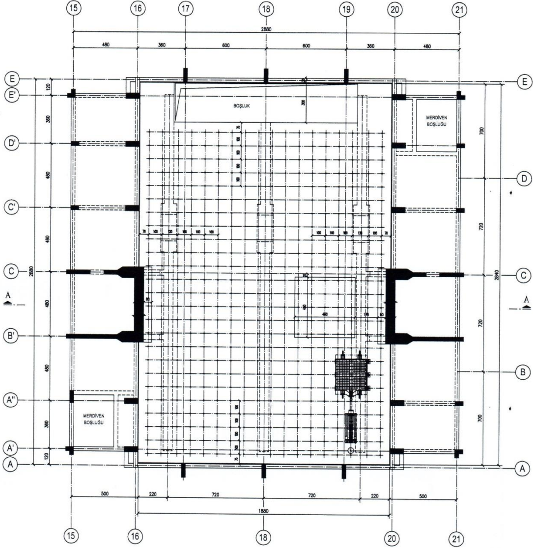
RÖLÖVE ZEMİN KAT PLANI 1/100
